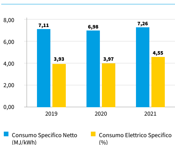
Grafico 13: Consumi energetici
