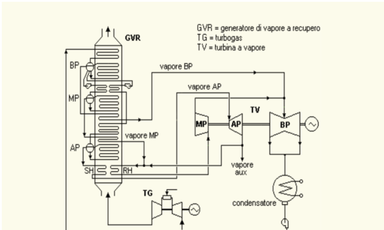
Figura 8: Schema semplificato dell'impianto
