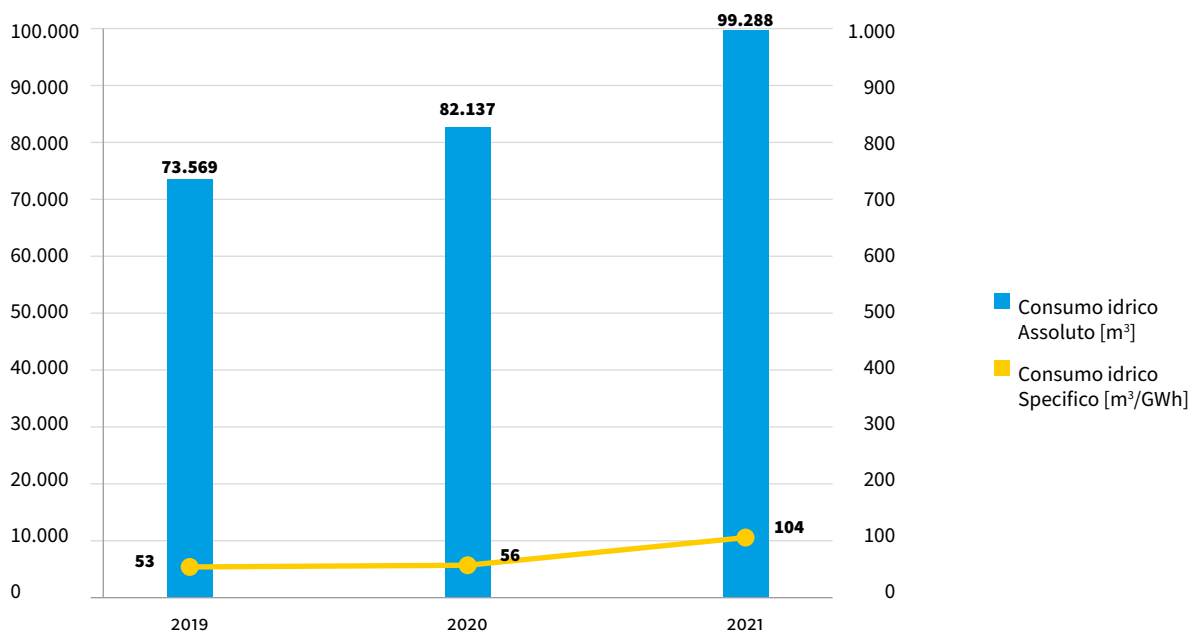
Grafico 9: Consumi idrici
