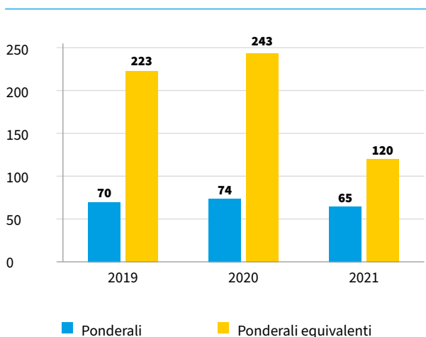
Grafico n. 3: Confronto delle emissioni ponderali di NO x con il valore limite equivalente
