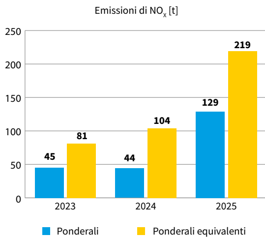
Grafico 3: Confronto delle emissioni ponderali di NO x con il valore limite equivalente
