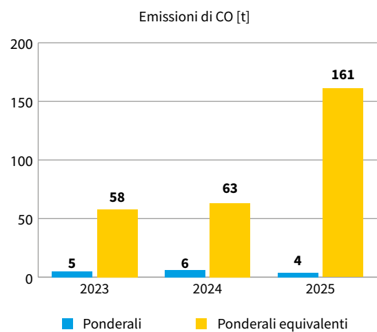
Grafico 4: Confronto delle emissioni ponderali di CO con il valore limite equivalente
