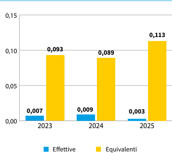
Grafico 6: Emissioni specifiche di CO [g/kWh]
