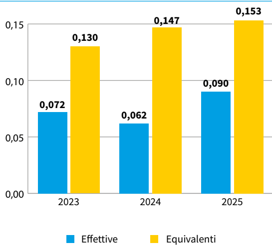
Grafico 5: Emissioni specifiche di NO x [g/kWh]
