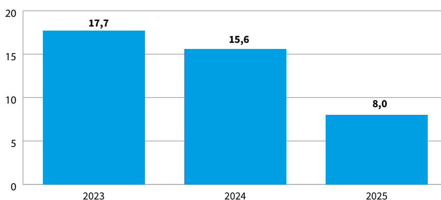
Grafico 15: Biodiversità [m²/GWh]
